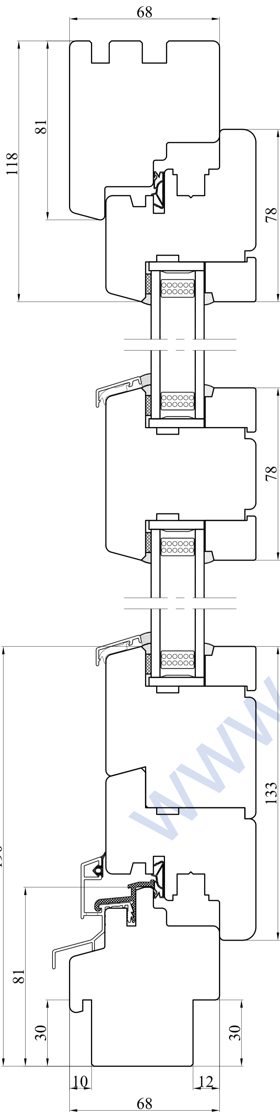
Przekrój A-A
