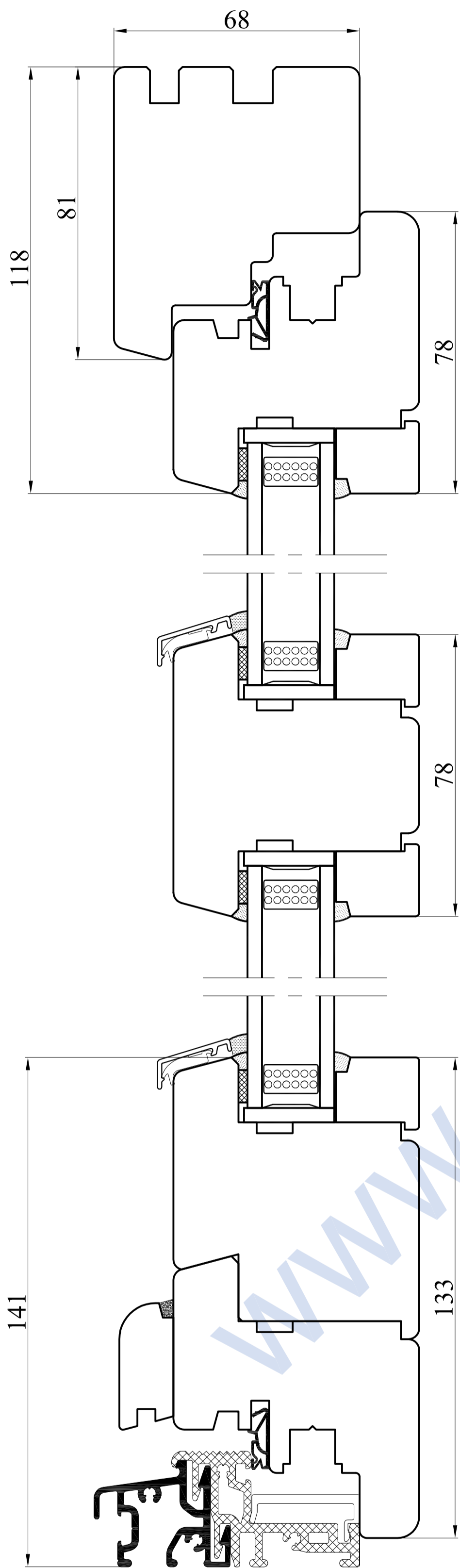
Przekrój A-A
