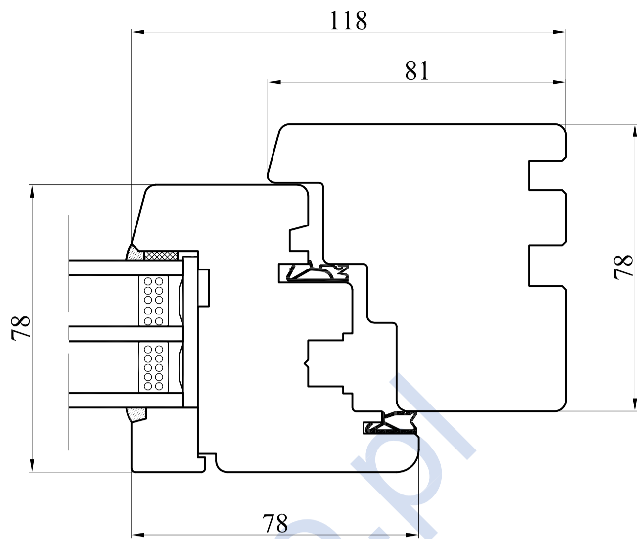
Przekrój B-B
