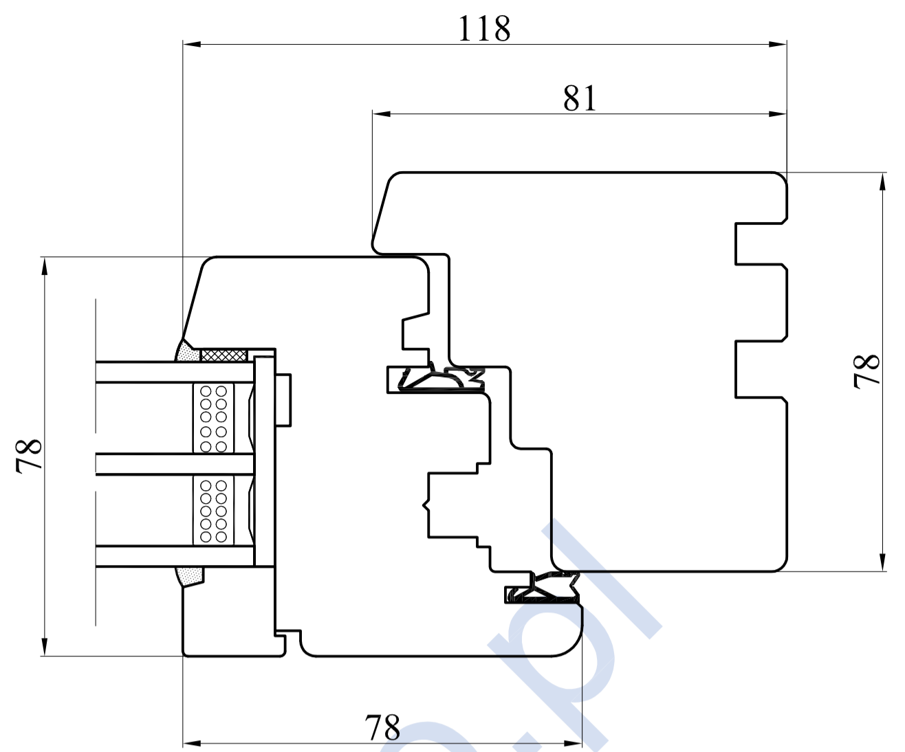
Przekrój B-B
