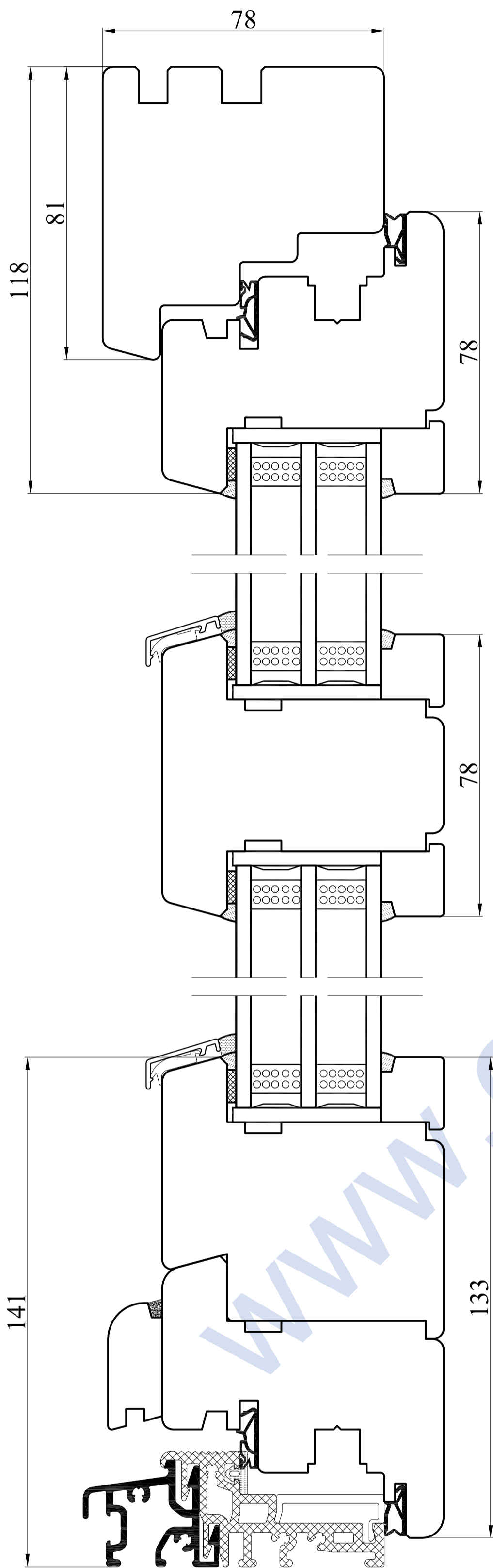
Przekrój A-A
