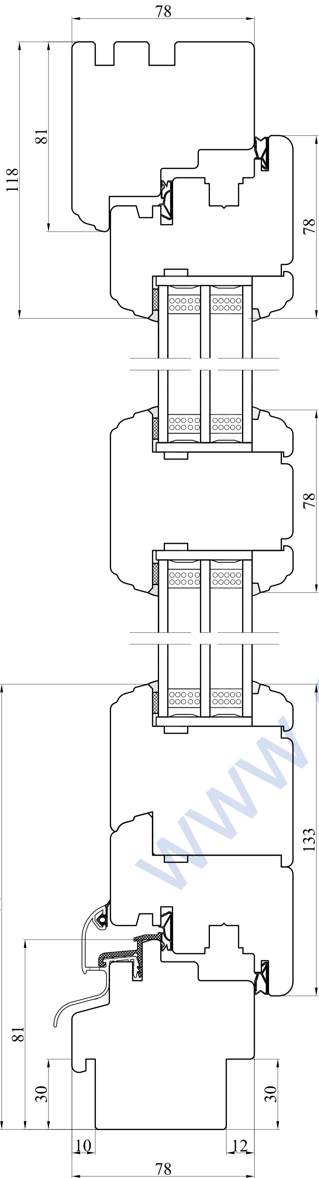
Przekrój A-A
