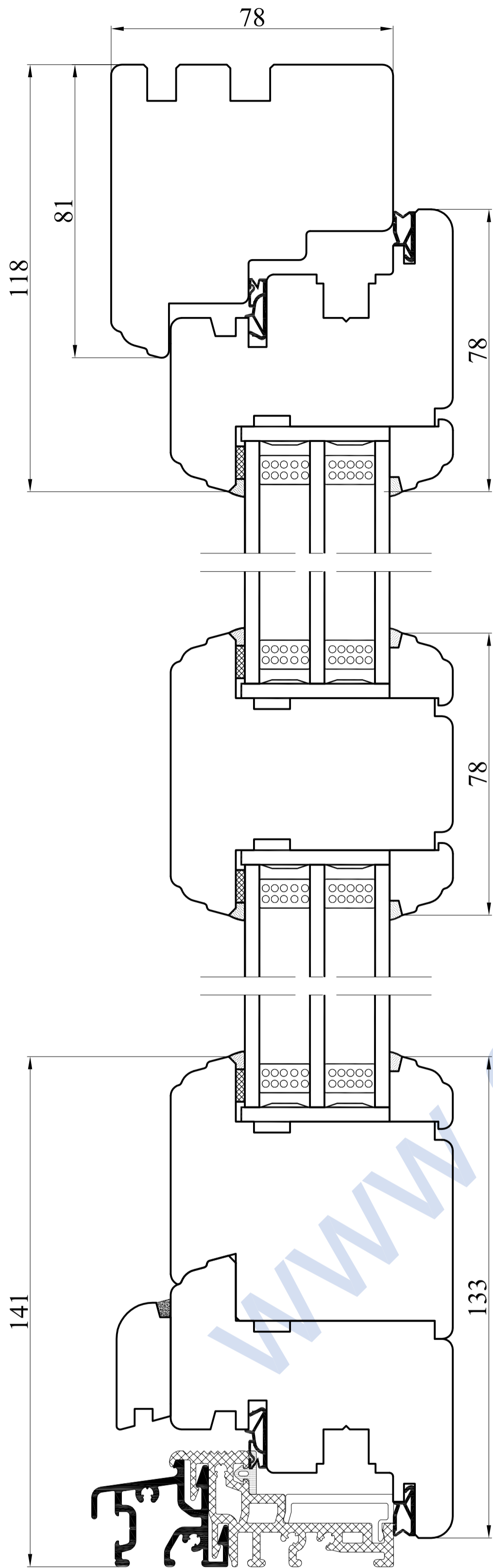
Przekrój A-A
