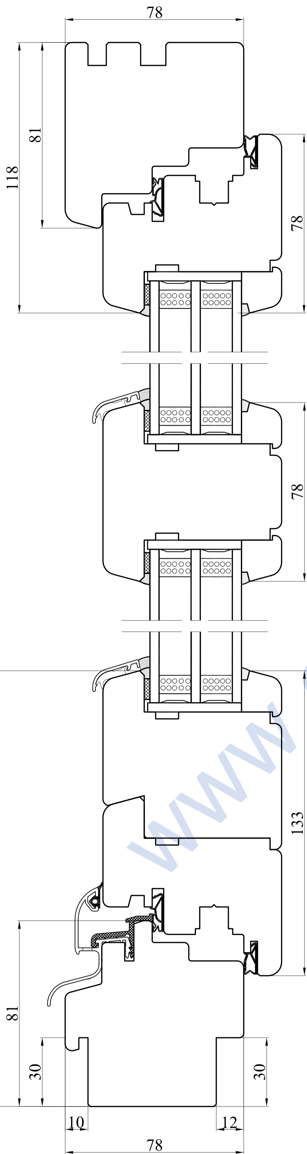
Przekrój A-A
