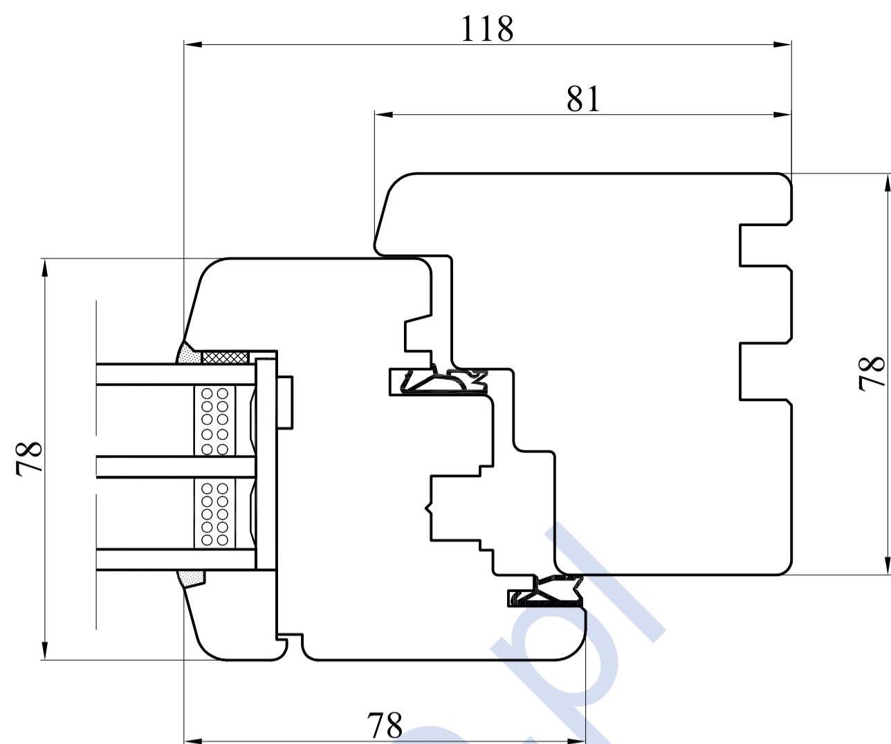
Przekrój B-B
