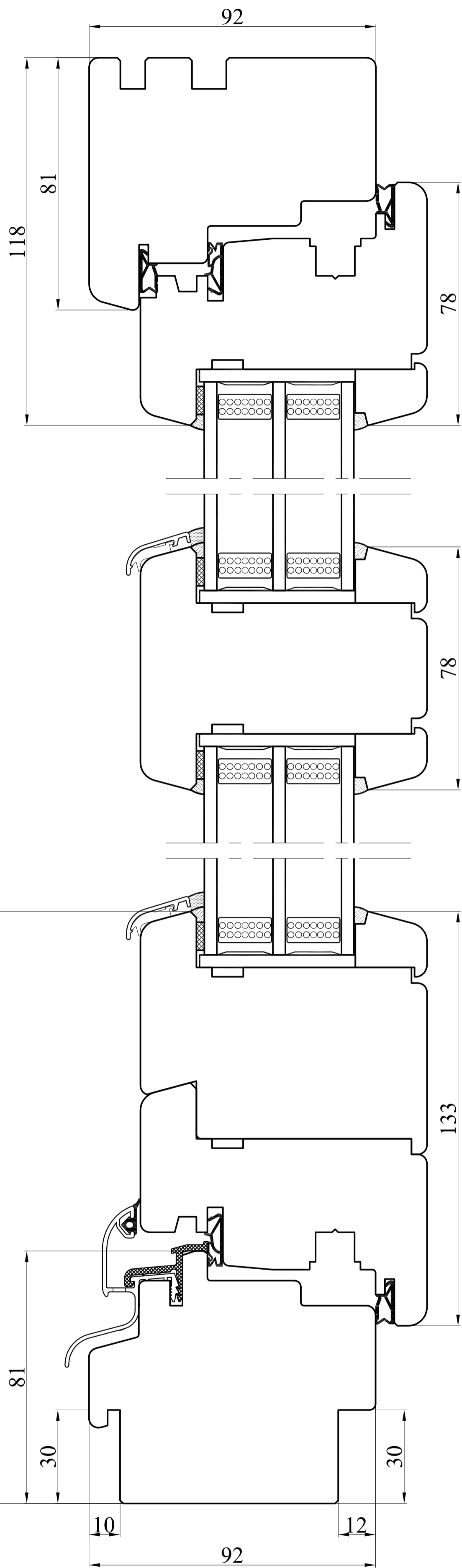
Przekrój A-A
